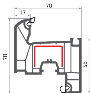
стулка
