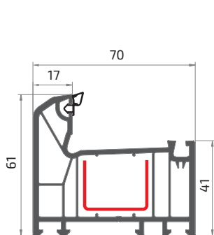
рама
