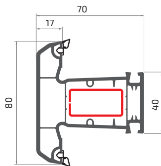
імпост
