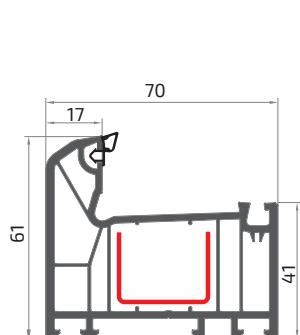
рама
