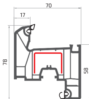
стулка
