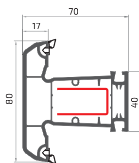
імпост
