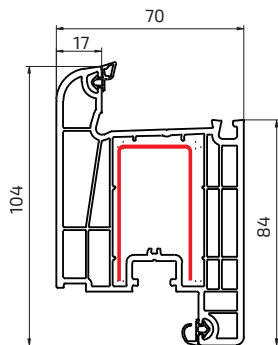
стулка внутрішнього відкриття
