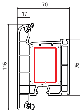
стулка зовнішнього відкриття
