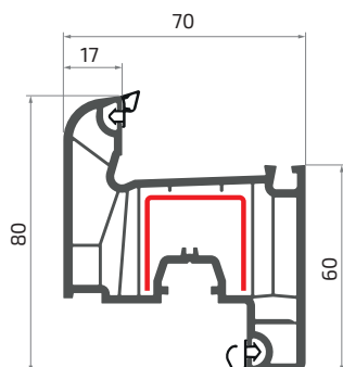
стулка
