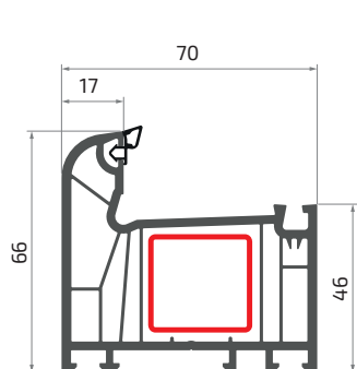
рама
