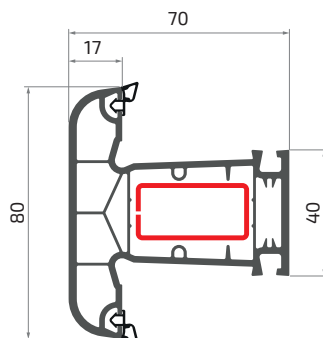
імпост
