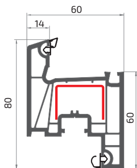
стулка
