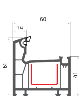
рама
