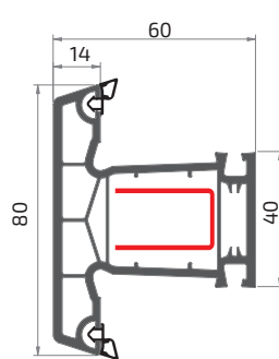
імпост
